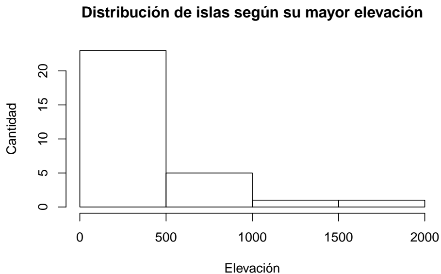
Gráfica 5.4: Histograma para la distribución de islas según su mayor elevación
